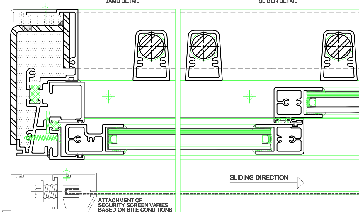
4 JAMB DETAIL
