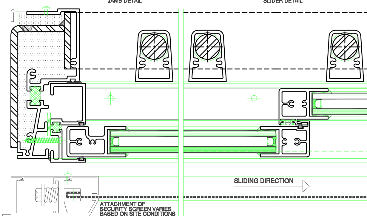
4 JAMB DETAIL
